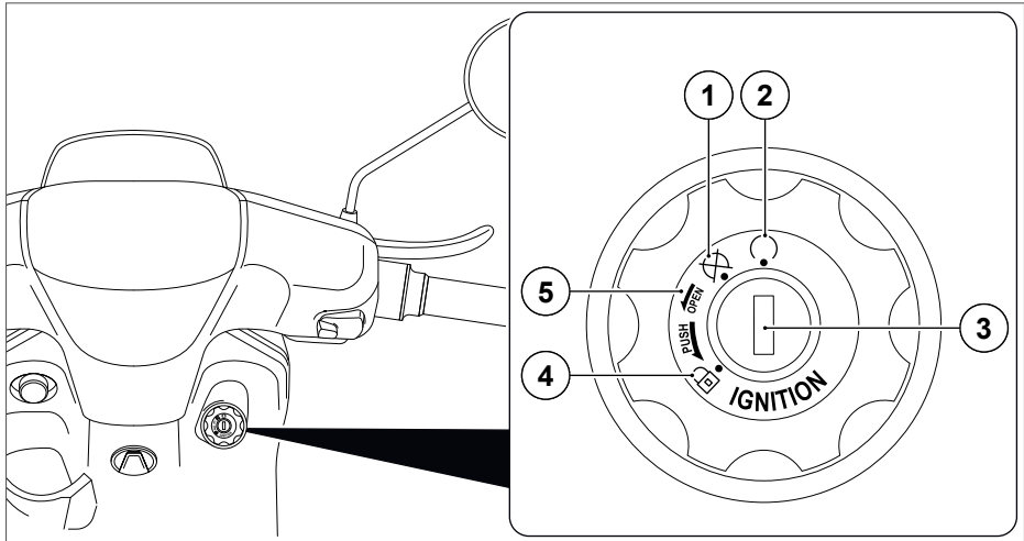
Abb. 7 Zündschloss (Beispieldarstellung)
